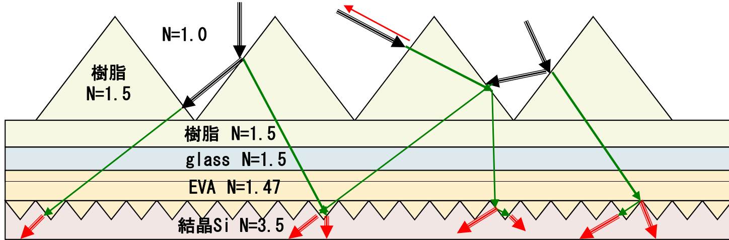
④ 片面SOH-1構造 ( Si texture 頂角90度固定)
