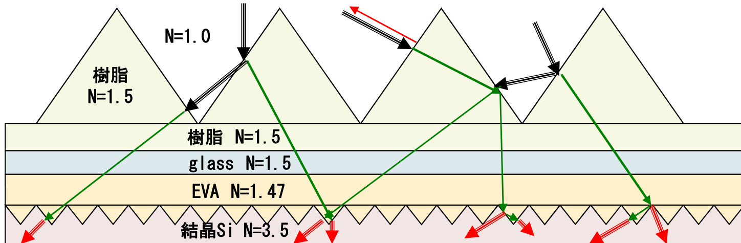
⑤ 片面SOH-1構造 ( Si texture 頂角可變)
